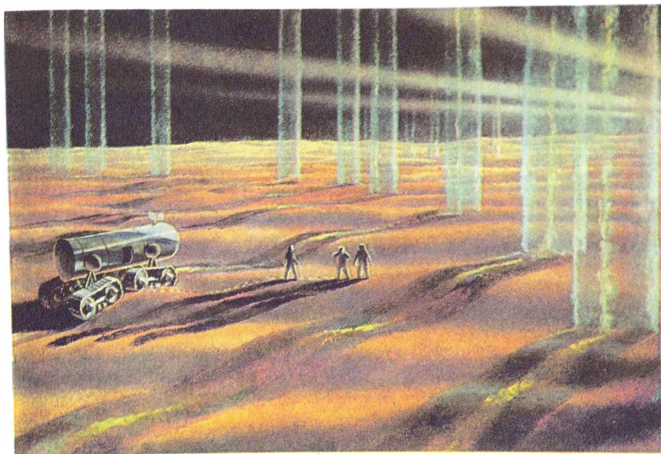
А. Соколов, Еще одна загадка Марса — Долина Призраков.
