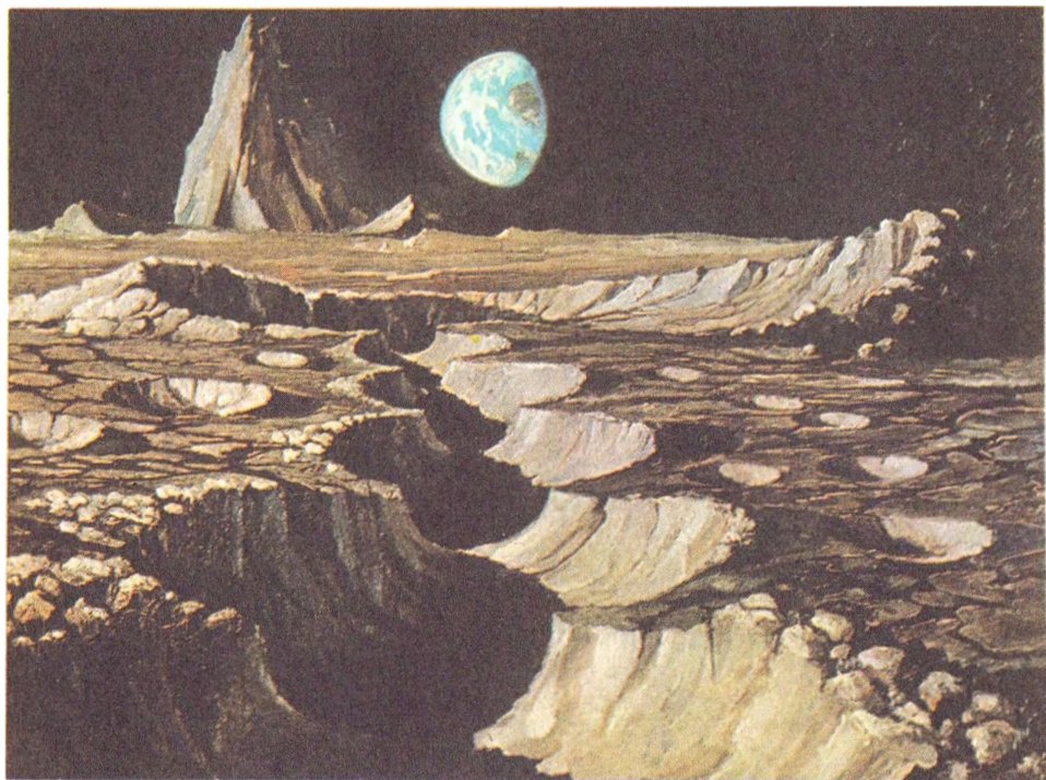
А. Леонов, Кратерные цепочки на Луне.
